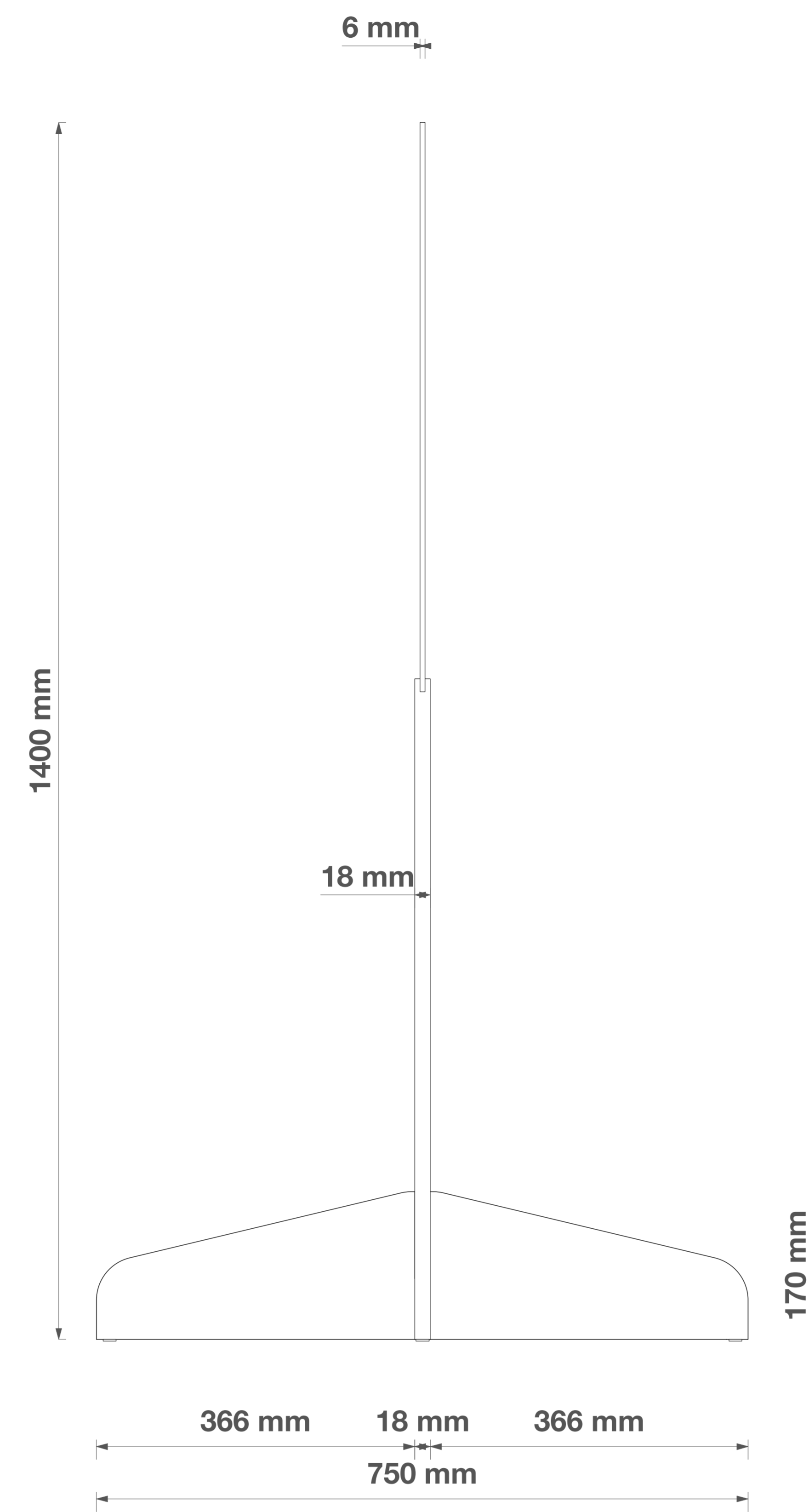
ANSICHT SEITE
